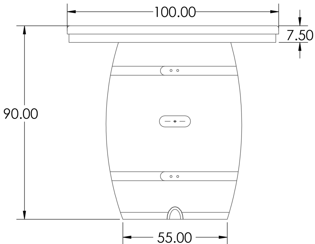
Elülső nézet
