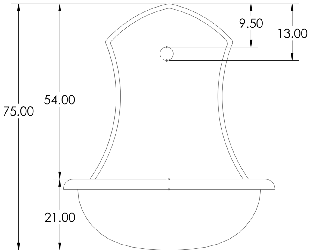
Elülső nézet
