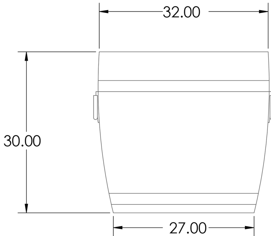
Elülső nézet
