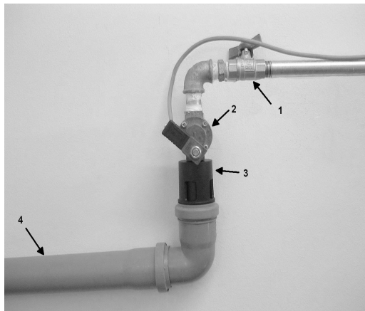
Abbildung 3: Montagebeispiel Rohrunterbrecher
