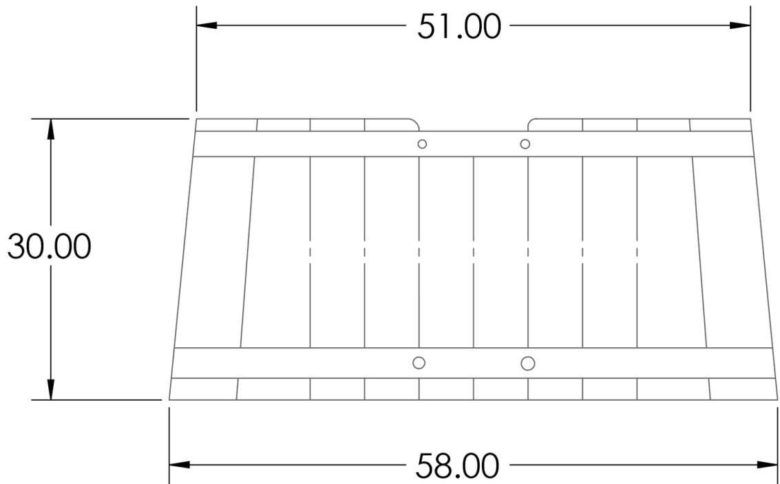
Elülső nézet
