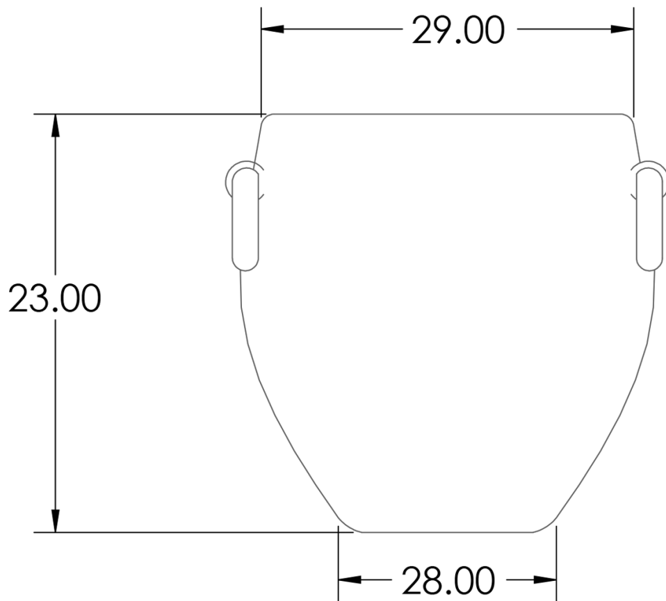
Elülső nézet
